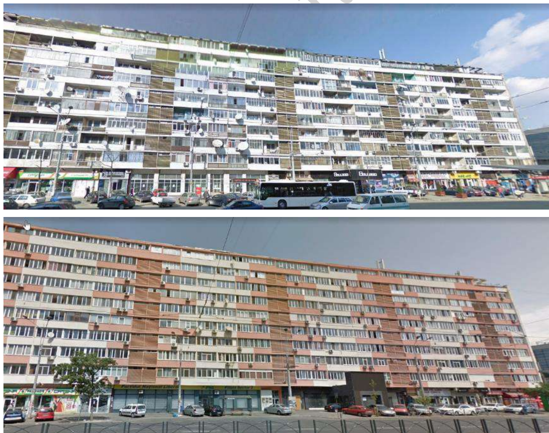
Figura 7.13 Clădire cu structura cu parter flexibil din beton armat amplasată în București, construită înainte de 1977 (înainte și după reabilitarea termică) (sursa: google maps)
